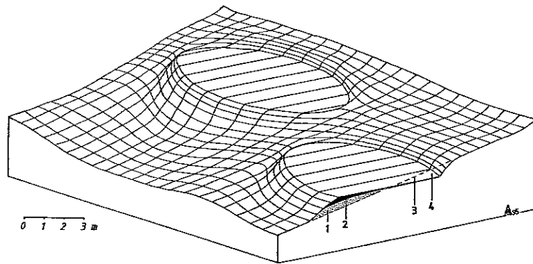
Abb. 7: Kohlenmeilerplatz, Doppelplatte. Schematische Darstellung der typischen Geländesituation in Hanglage mit runder Verebnung von etwa 8 m Durchmesser, talseitiger Auffüllung (1), holzkohlereicher Schicht (2), ehemaligem Hangverlauf (3, gestrichelt) und bergseitiger Abgrabung (4).
