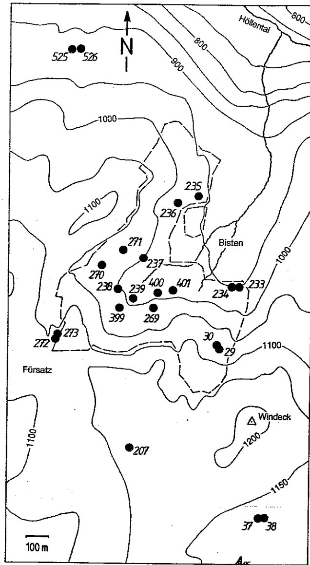
Abb. 4: Untersuchungsgebiet Bisten-Windeck am Rande des Höllentales. Die 22 bearbeiteten Meilerplätze liegen im Bistenkar, an den steilen Karwänden und auf den angrenzenden Hochflächen. Gestrichelt: Kartierungsfläche (Vegetationskarte Bistenkar, Abb. 14).
