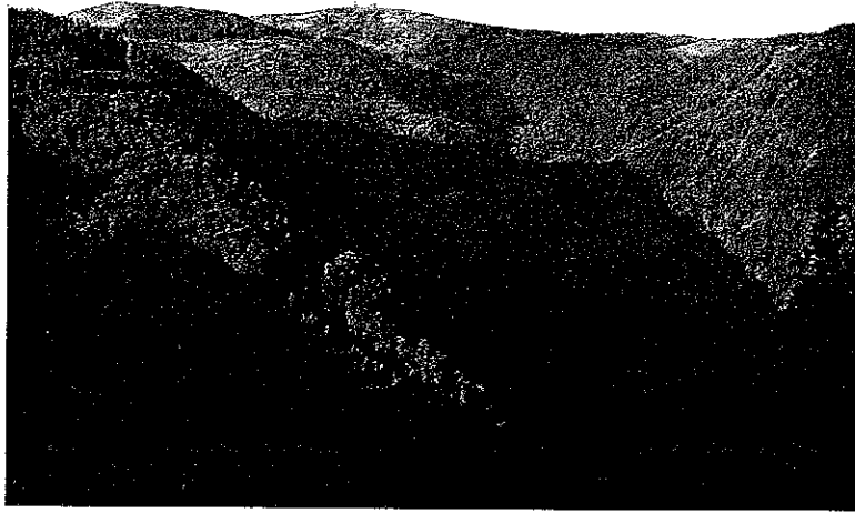
Abb. 2: Das tief eingeschnittene Zastlertal und die flacheren Kamm- und Kuppenlagen unmittelbar nördlich des Feldbergs im Südschwarzwald: im Hintergrund links mit Schneeflecken und Gebäuden der Hauptgipfel (1493 m), ganz links der Baldenweger Buck (1461 m), rechts der teilweise bewaldete Immisberg (1373 m) mit seinem waldfreien, von Weideland bedeckten Nordhang. Hier liegen die höchsten bearbeiteten Meilerplätze (1350 m); die tiefsten befinden sich ziemlich genau in der Bildmitte im Talgrund nahe der Schattengrenze auf gut 1000 m. Die Kartierungsfläche „Schonwald Zastler Loch“ erstreckt sich von dort zum Baldenweger Buck hinauf. 29.6.1988.
