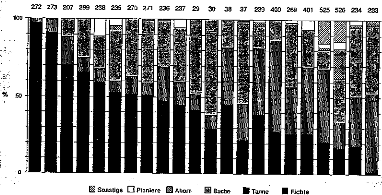
Abb. 19: Untersuchungsgebiet Bisten/Südschwarzwald. Ergebnisse der Holzkohlenanalyse von 22 Meilerplätzen, angeordnet nach benachbarter/standörtlich-topographisch ähnlicher Lage im Gelände, links auf der Hochfläche über 1100 m beginnend hinab ins westliche Bistenkar und von dort über die zentralen zu den östlichen und tiefsten Plätzen hin (unter 1000 m; vgl. Abb. 4). Als Pioniere wurden Eberesche (Pomoideae), Birke, Weide und Pappel zusammengefaßt, als Sonstige Erle, Esche und Ulme. Die in der Holzkohle angetroffene Artenkombination verändert sich ± fein abgestuft von Fichten-beherrschten Proben zu Buchen- oder Tannen-dominierten mit den niedrigsten Fichtenwerten.
