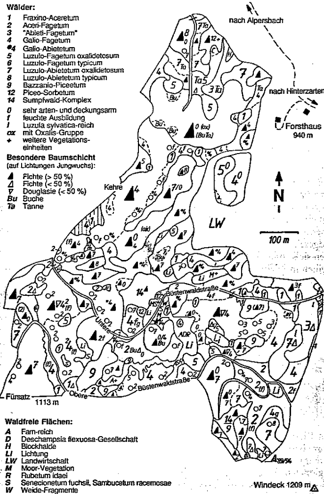
Abb. 14: Vegetationskarte Bistenkar. Die 48 ha große Kartierungsfläche im Bistenkar erstreckt sich über 200 Höhenmeter vom Karboden bei 950 m auf etwa 1150 m am Windeck. Die Wälder werden hier überwiegend von Fichten-dominierten Beständen aufgebaut, die nach der Bodenvegetation verschiedenen Waldgesellschaften nährstoffreicher Standorte zugeordnet wurden (2, 4, 7, 8), an Aushagerungsstandorten auch dem Luzulo-Abietetum (7, 8). (Lage der Kartierungsfläche vgl. Abb. 4; weitere Erläuterungen in Kap. 2.5 u. 3.2)
