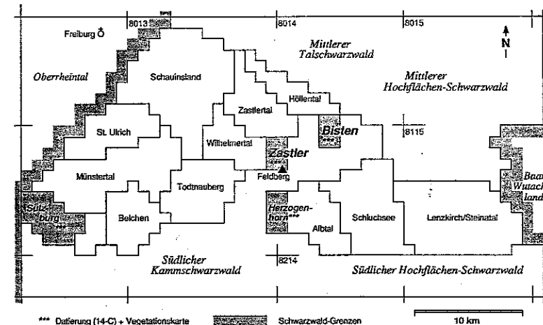
Abb. 1: Lage der Untersuchungsgebiete Zastler und Bisten im Südschwarzwald im Übergangsbereich der verschiedenen Naturräume: im Westen Mittlerer Tal- und Südlicher Kamm-Schwarzwald (rhenanisch), im Osten Mittlerer und Südlicher Hochflächen-Schwarzwald (danubisch). Gezeichnet sind weitere Untersuchungsgebiete sowie die Ausschnitte der Topographischen Karten 1:25000 mit ihren Nr. (vierstellige Ziffern). Vom Südabfall des Feldbergs (Herzogenhorngebiet) und aus dem alten Bergbaurevier Sulzburg am Schwarzwald-Westrand liegen ebenfalls holzkohleanalytische Untersuchungen an Meilerplätzen vor (LUDEMANN 1994b, 1996).
