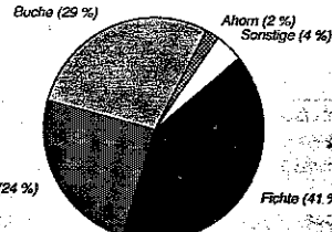
Abb. 16: Untersuchungsgebiet Bisten/Südschwarzwald. Anteil der nachgewiesenen Arten in der Holzkohle von 22 spätmittelalterlich-frühneuzeitlichen Meilerplätzen. Als Sonstige wurden Erle, Eberesche (Pomoideae), Esche, Birke, Weide, Ulme und Pappel zusammengefaßt. Datenbasis: 2347 Stücke = 100%. Die Plätze liegen zwischen 910 und 1150 m ü. NN, durchschnittlich gut 1000 m hoch.
