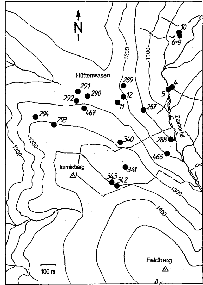
Abb. 3: Untersuchungsgebiet Zastler/Südschwarzwald unmittelbar nördlich des Feldbergs (1493 m). Die 23 bearbeiteten Meilerplätze liegen auf einem flachen Höhenrücken der danubischen Altlandschaft und im tief eingeschnittenen Zastlertal. Gestrichelt: Westteil der Kartierungsfläche (Vegetationskarte Schonwald „Zastler Loch“, Abb. 13)
