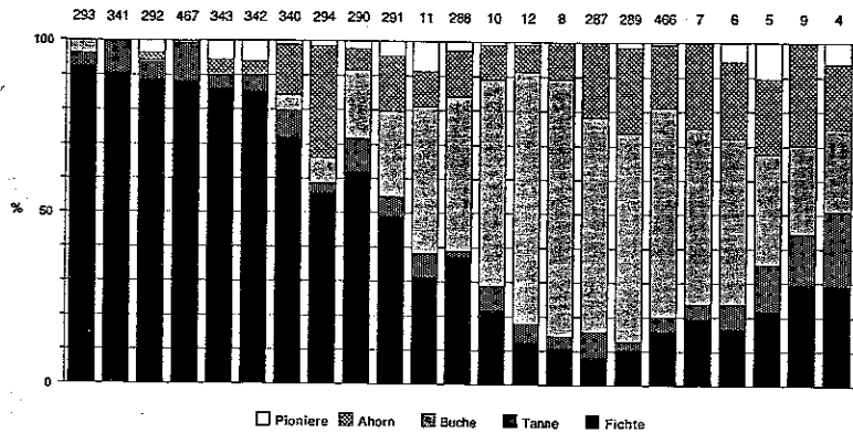
Abb. 18: Untersuchungsgebiet Zastler/Südschwarzwald. Ergebnisse der Holzkohlenanalyse von 23 Meilerplätzen, angeordnet nach benachbarter/standörtlich-topographisch ähnlicher Lage im Gelände, links bei den hohen Kammlagen über 1300 m beginnend, über die Steilhänge des Zastlertales nach rechts zum Talgrund hin (unter 1100 m; vgl. Abb. 3). Als Pioniere wurden Eberesche (Pomoideae) und Weide zusammengefaßt. Die in der Holzkohle angetroffene Artenkombination verändert sich fein abgestuft von den Fichten-beherrschten Proben, ohne und mit deutlicher Ahornberei-tigung, über Buchen-dominierte und Ahorn-reiche hin zu Proben mit ziemlich ausgeglichenem Verhältnis der vier Hauptbaumarten und den höchsten Tannenwerten bei wieder ansteigendem Nadel-baumanteil.
