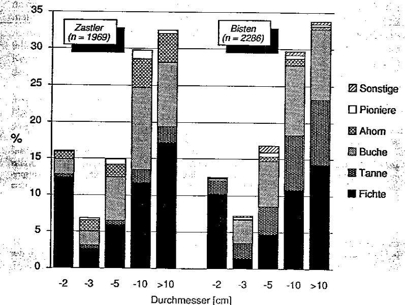
Abb. 20: Verteilung der Holzkohlenstücke auf Durchmesserklassen für das Gesamtmaterial der Untersuchungsgebiete Zastler und Bisten im Südschwarzwald. n Stückzahl/Datenbasis (= 100%). Als Pioniere wurden Eberesche (Pomoideae), Birke, Weide und Pappel zusammengefaßt, als Sonstige Erle, Esche und Ulme. Zum größten Teil wurde starkes Holz (> 5 cm Durchmesser) verwendet. Ein zweites, niedriger „Gipfel“ zeigt sich für Fichte beim schwächsten Holz, worin die Nutzung von Fichtenzweigen als Abdeckmaterial der Meiler zum Ausdruck kommt.
