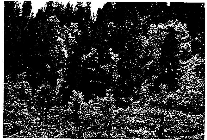
Abb. 21: In den Hochlagen-Fichtenbeständen in feuchten, nährstoffreichen Mulden ausklingender Bergahorn-Buchenwald (Aceri-Fagetum) am Feldberg/Südschwarzwald. Diese Bestandes-Situation wird durch die Meilerplätze K 294 und K 340 dokumentiert (Abb. 18), die mit deutlicher Beteiligung von Ahorn bei vorherrschender Fichte eine vermittelnde Stellung zwischen den Laubholz-reichen Plätzen der tiefer liegenden Steilhänge und den Fichten-reichsten Plätzen der höchsten Kammlagen einnehmen. 6.1985.
