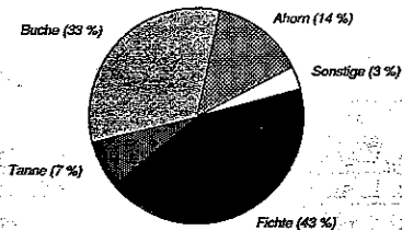
Abb. 15: Untersuchungsgebiet Zastler/Südschwarzwald. Anteil der nachgewiesenen Arten in der Holzkohle von 23 spätmittelalterlich-frühneuzeitlichen Meilerplätzen. Als Sonstige wurden 80 Stücke von Eberesche (Pomoideae) und 5 von Weide zusammengefaßt. Datenbasis: 2700 Stücke = 100%. Die Plätze liegen zwischen 1030 und 1350 m ü. NN, durchschnittlich knapp 1200 m hoch.
