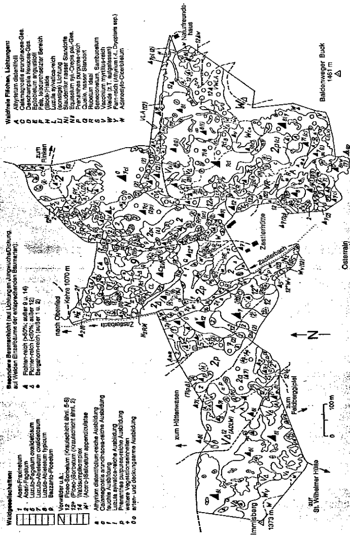
Abb. 13: Vegetationskarte Schonwald „Zastler Loch“ (aus LUDEMANN 1992b). Die 60 ha große Kartierungsfläche erstreckt sich über 350 Höhenmeter zwischen 1070 m im Norden am Zasterbach und 1420 m im Südosten beim Baldenweger Buck. An den steilen Hängen und im Talgrund des Zasterbaches herrschen kraut- und hochstaudenreiche Bergahorn-Buchenwälder vor (2, Aceri-Fagetum). Die flachen Höhenrücken am Immisberg und am Baldenweger Buck (linker und rechter Teil der Karte) werden von Fichtenbeständen besiedelt, die nach der Bodenvegetation dem Luzulo-Abietetum (7, 8) zuzuordnen sind. (Lage der Kartierungsfläche vgl. Abb. 3; weitere Erläuterungen in Kap. 2.5 u. 3.2)
