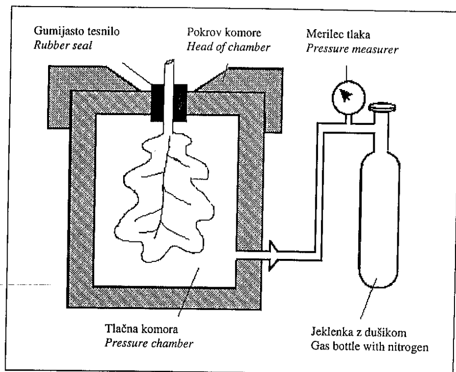
Slika 2: Shematski prikaz merjenja vodnega potenciala
