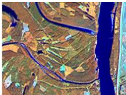
Buvat, Keszeges-tó ER, SPOT4 - FÖMI úrfotótérkép Buvat, Keszeges-tó Erdőrezervátum FÖMI (Eurimage) 1999 er29_30.JPG
